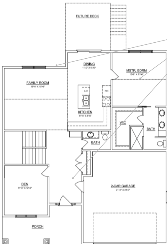
① FIRST FLOOR PLAN 10.00.10.01.01
