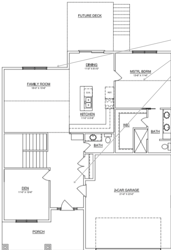
① FIRST FLOOR PLAN 10.00.10.00.00
